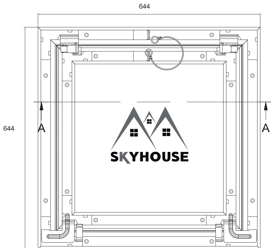
TAPA INSPECCION 60 x 60 cm
